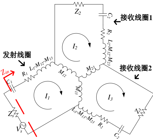
图 12 两线圈耦合系统等效电路模型
