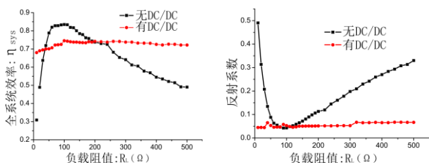
(a) 系统效率比较 (b) 系统反射系数比较
