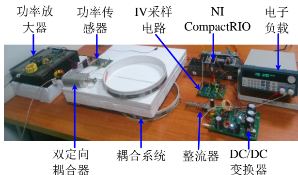
图 8 动态最优负载跟踪实验平台
