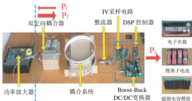
图 5 静态最优负载控制实验平台
