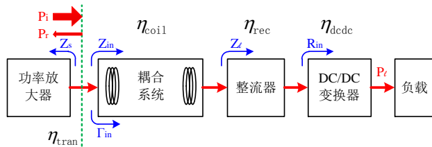
图 1 无线电能传输系统框图
