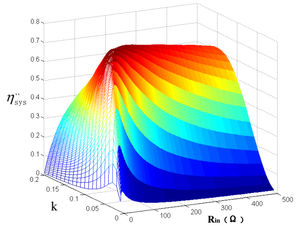
图 3 系统效率特性
