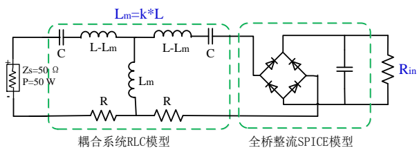
图 2 ADS 系统仿真电路模型
