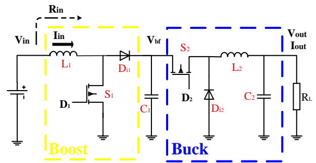
图 4 Boost-Buck 变换器拓扑
